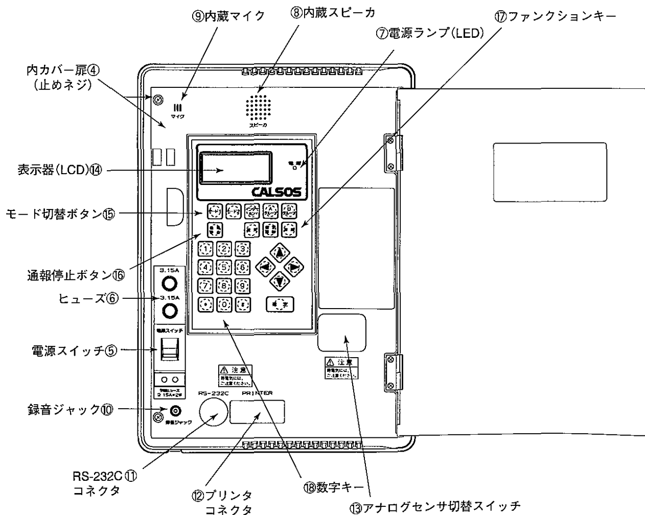
CS・D7通報装置(本体)内観図
