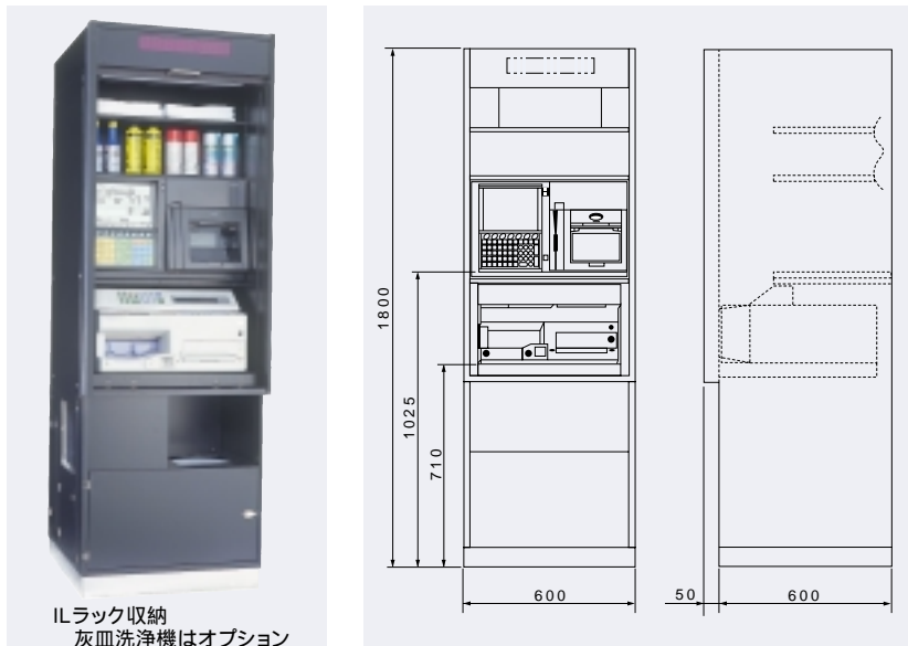
寸法図
